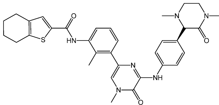
GDC-0834
