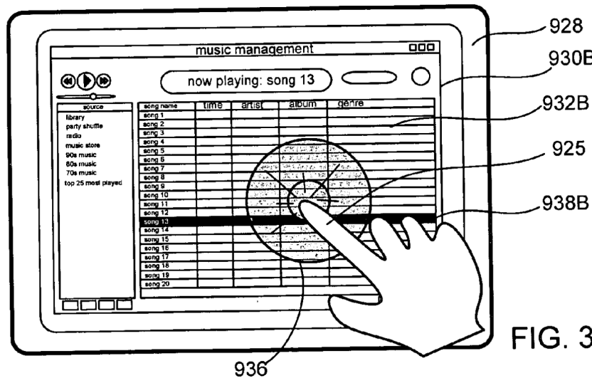
FIG. 35E
