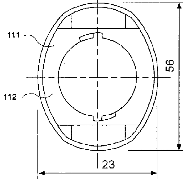
背面図
