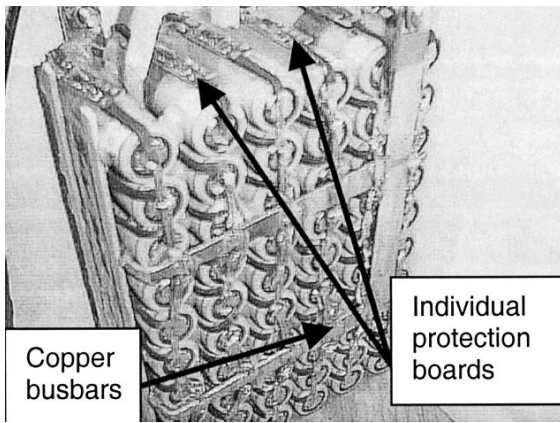
Fig. 3. Li-ion module (60 cells).
