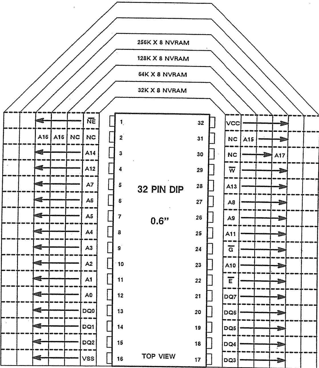
FUNCTION TABLE
