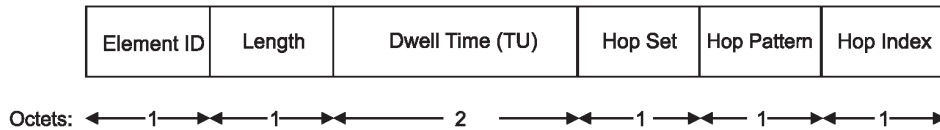
Figure 7-40—FH Parameter Set element format
