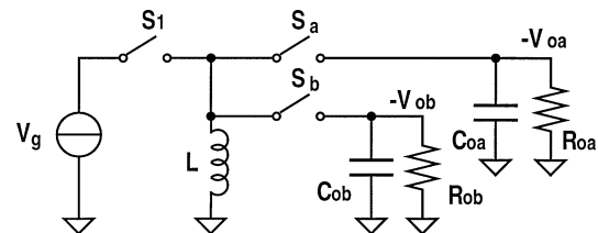
Fig. 11. SIDO flyback converter.
