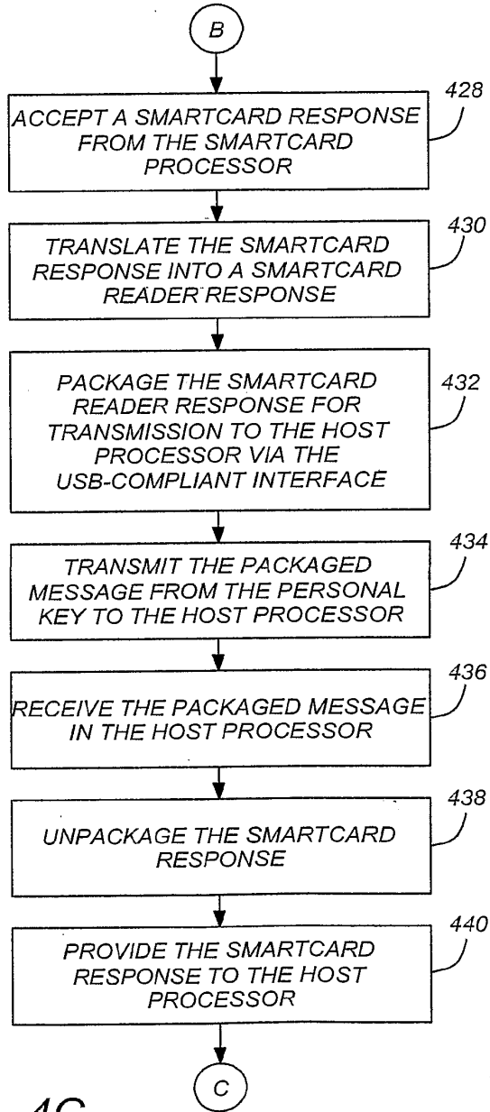
FIG. 4C
