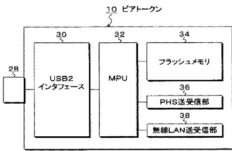
本発明によるピアトーンのハードウェア構成のブロック図
