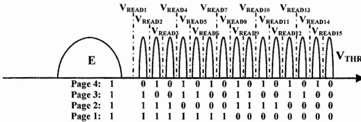
Fig. 16.32. 16LC coding
