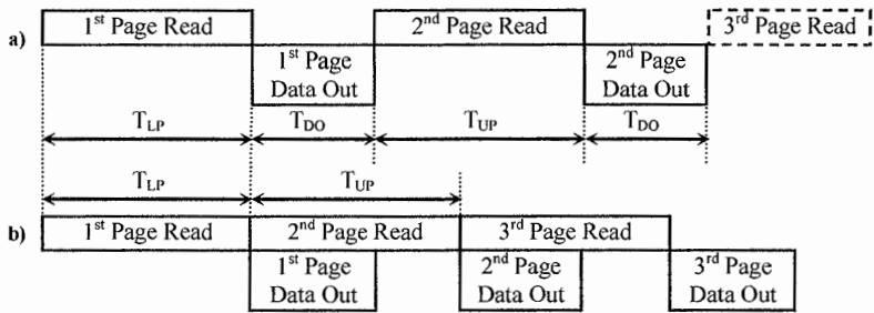
Fig. 10.12. Cache read
