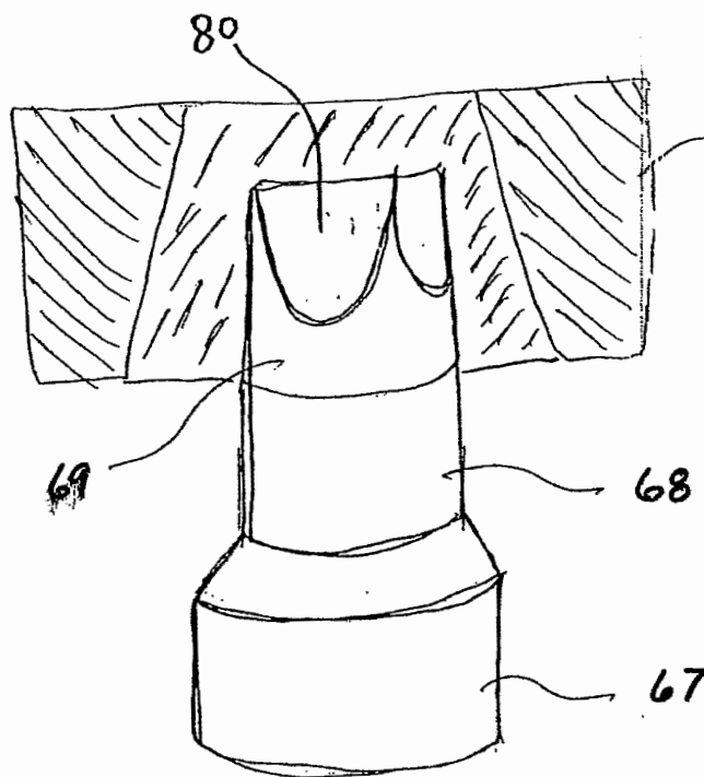
Fig. 6e
