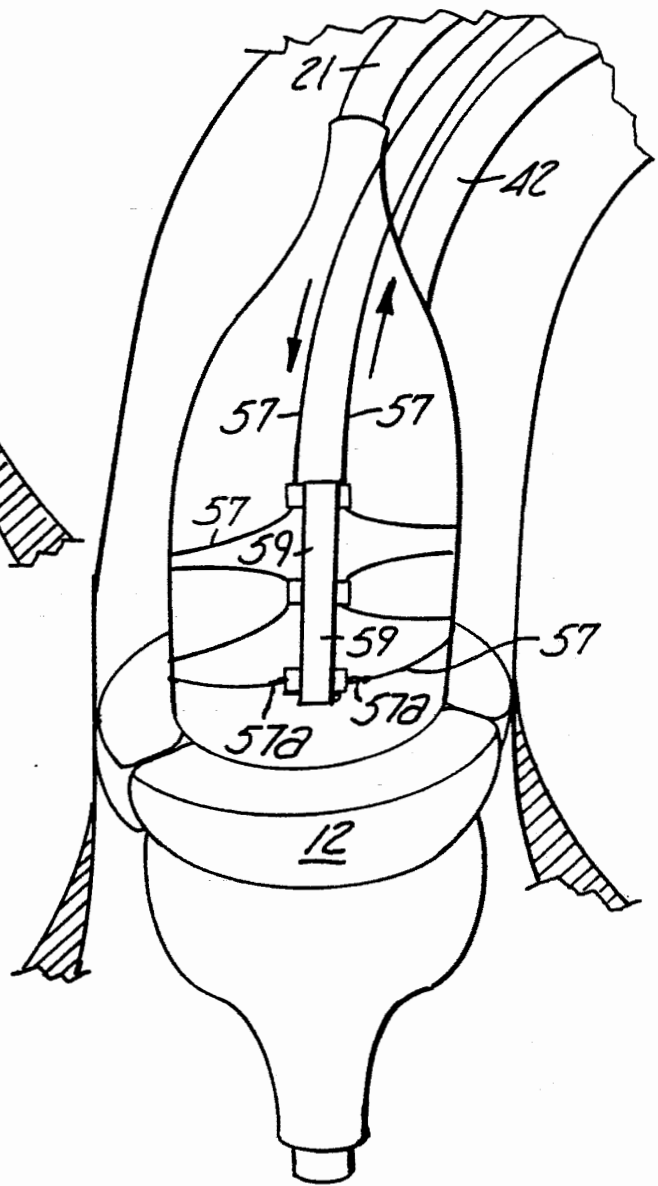
Fig. 16A
