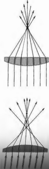
Figure 6.16 SA for a planar-convex lens.
