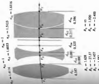
Figure 6.10 A Tessar.
