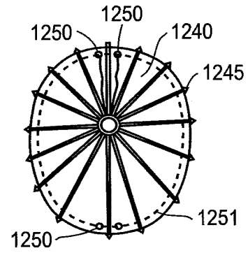
Section B - B' FIG. 30B
