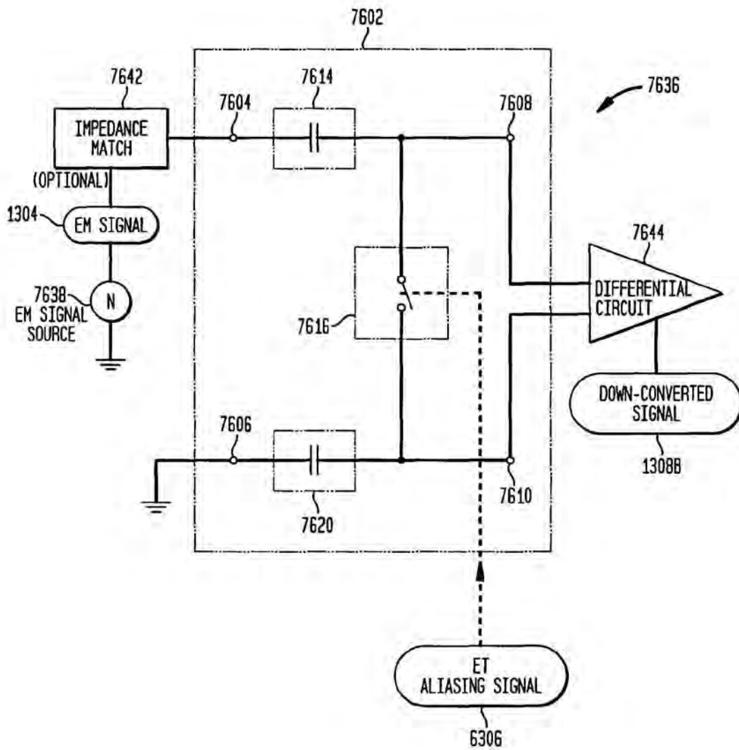
FIG. 76E EXAMPLE INPUT/OUTPUT CIRCUITRY
