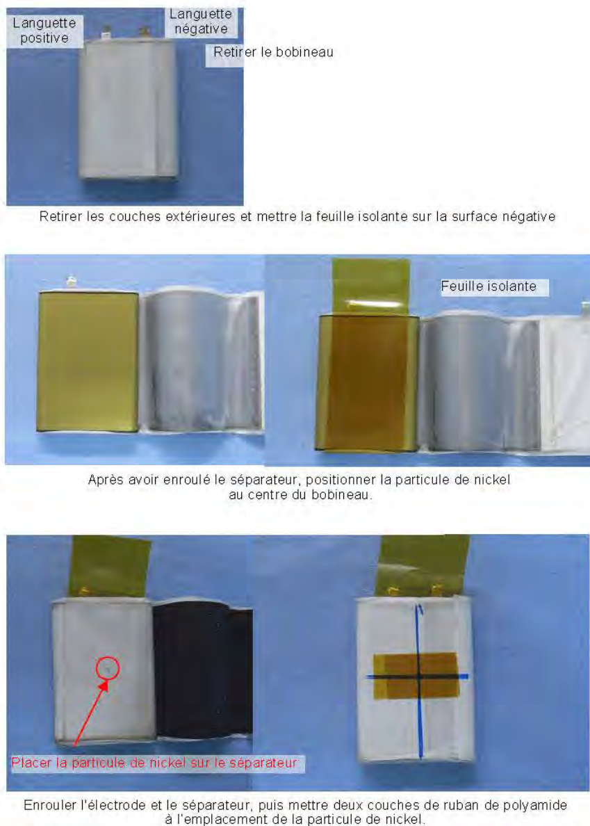
Figure A.9 – Démontage des éléments parallélépipédiques
