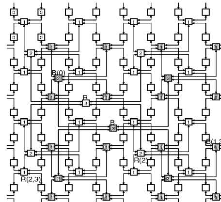
Fig. 4. Fat H-Tree
