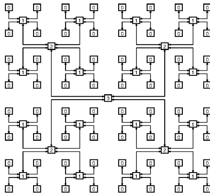
Fig. 3. H-Tree
