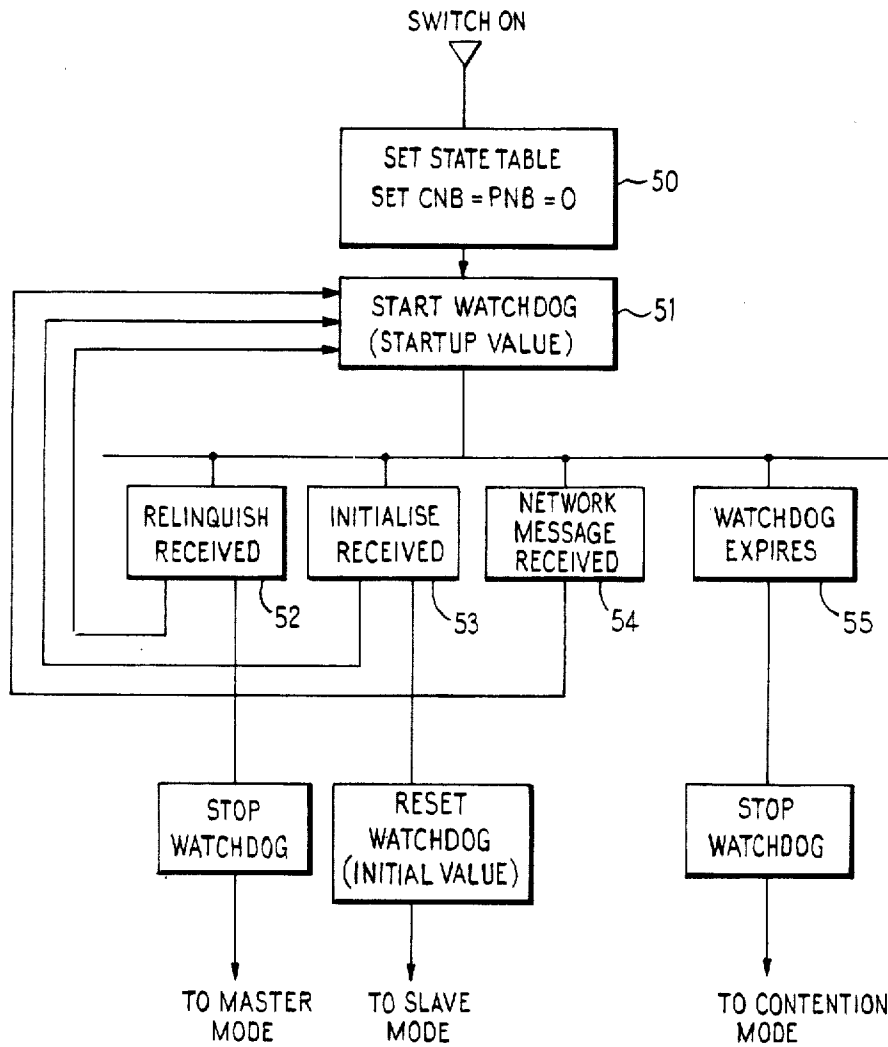
FIG. 5 STARTUP MODE
