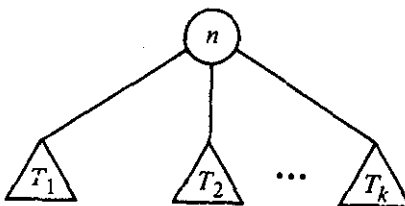
Fig. 3.4. Tree T .
