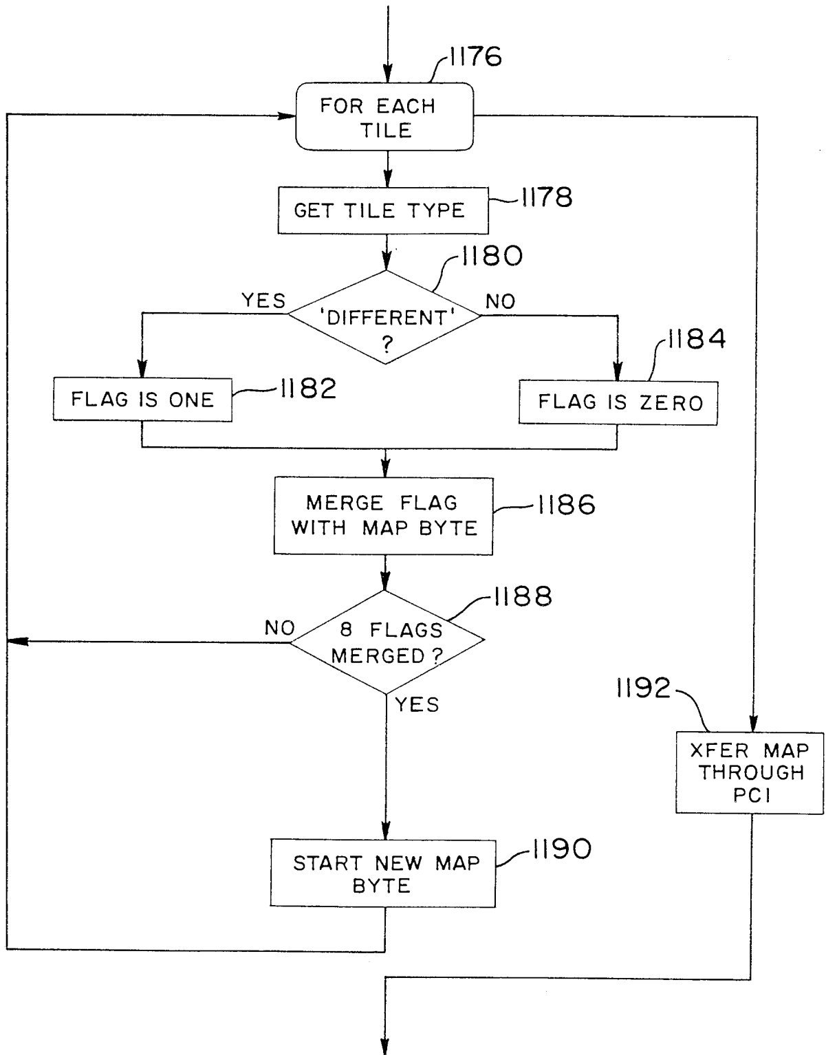
FIG. 39 A MAP GENERATOR
