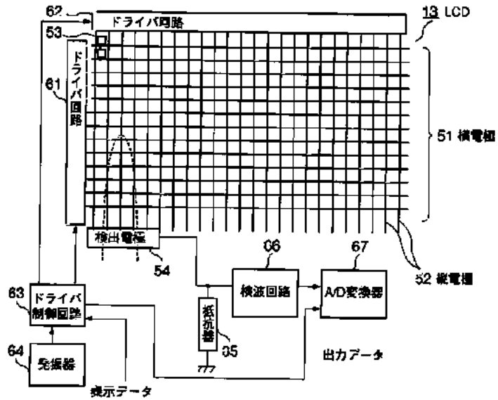
【図11】
