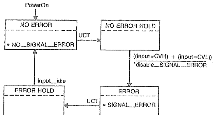
Fig 12-7 DTE PLS Input Function
