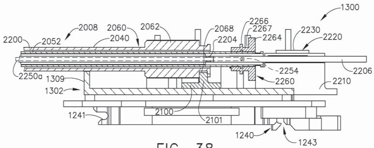
FIG. 37
