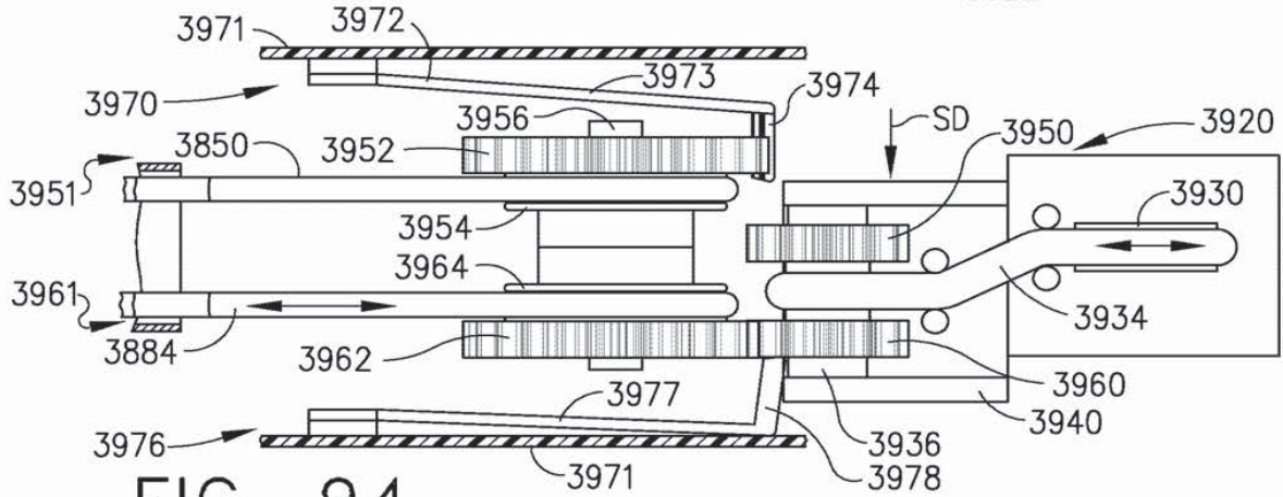
FIG. 94
