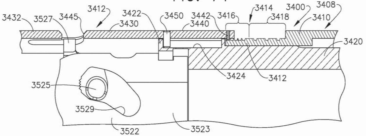
FIG. 72
