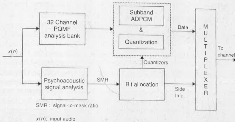
Figure 10.31. DTS-coherent acoustics (DTS-CA) encoding scheme.
