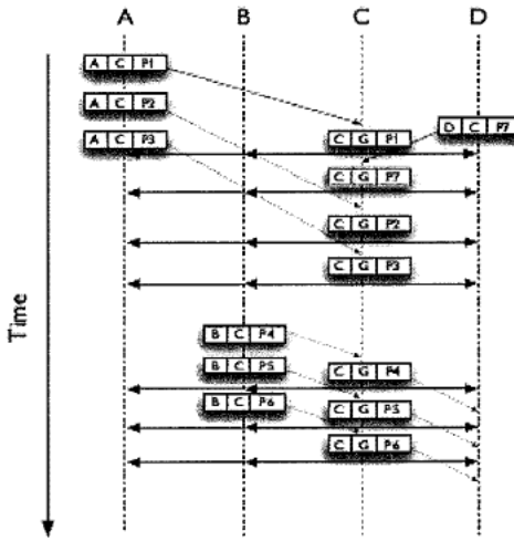
Dynseq Example Timeline
