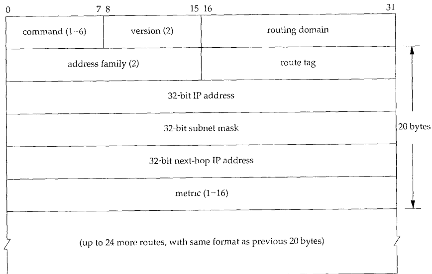
Figure 10.10 Format of a RIP-2 message.
