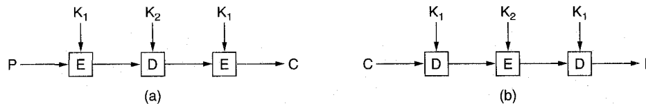
Fig. 7-9. Triple encryption using DES.
