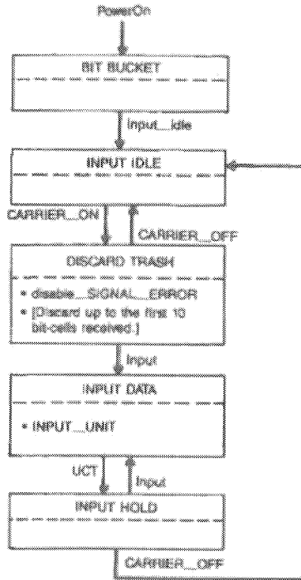
Fig 12-7 DTE PLS Input Function
