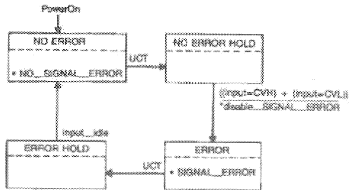
Fig 12-8 DTE PLS Error Sense Function
