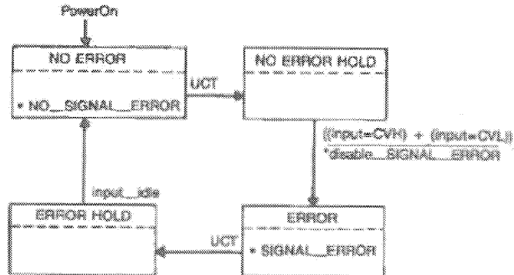
Fig 19-8 DTE PLS Error Sense Function
