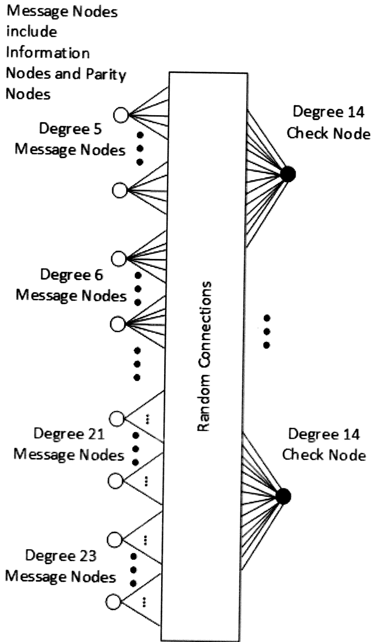
Tanner graph for Luby98's Code 14
