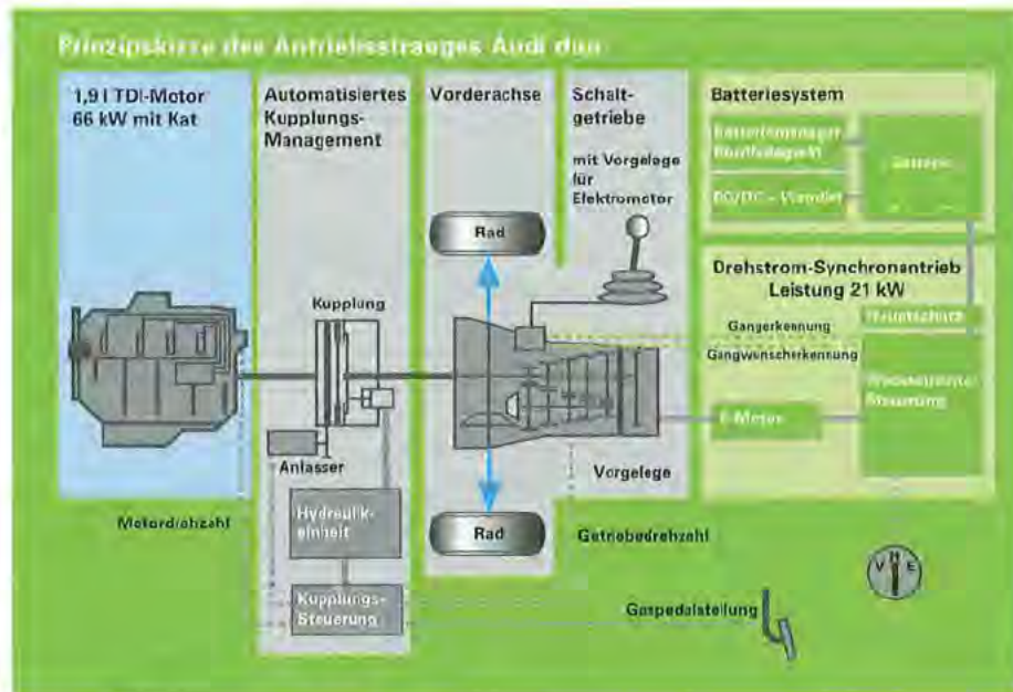
Bild 4: Prinzipdarstellung des Antriebsstrangs
