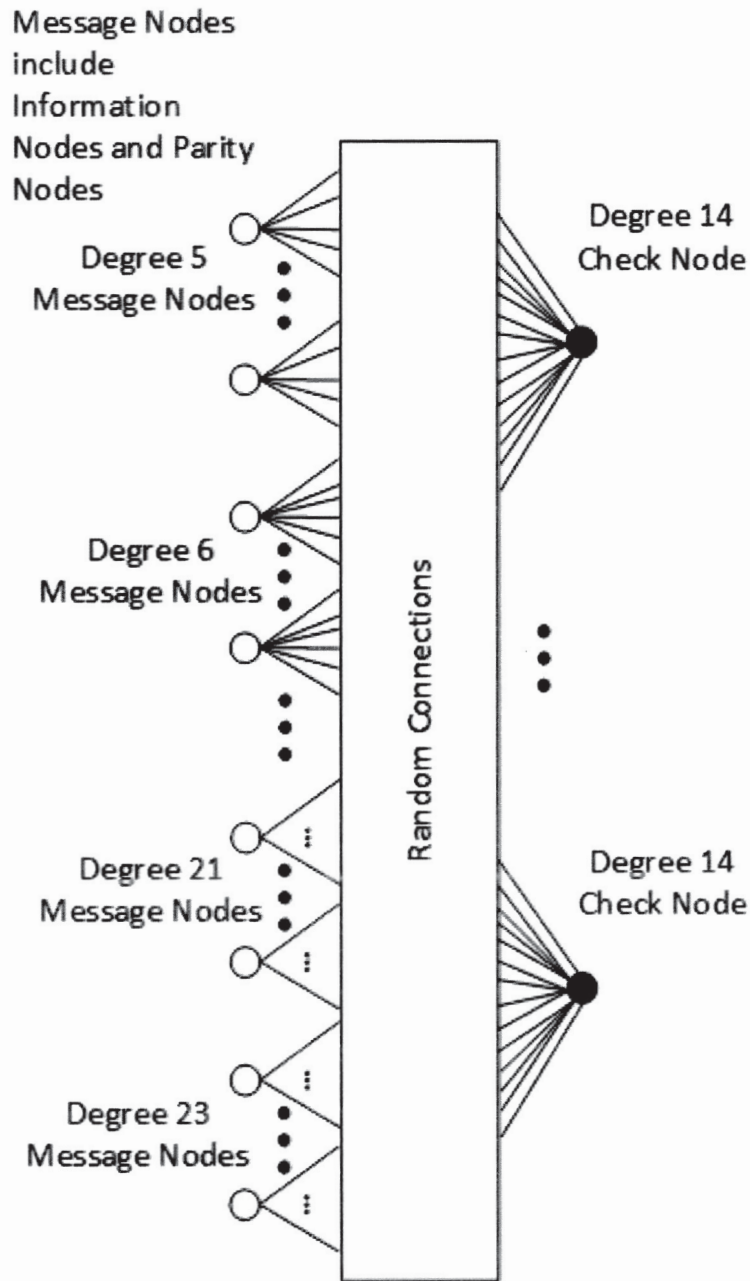
Tanner graph for Luby98's Code 14
