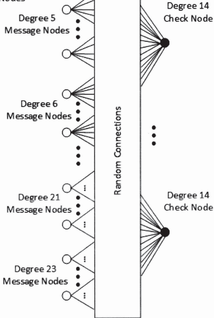
Tanner graph for Luby98's Code 14
