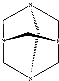
hexamethylenetetramine
