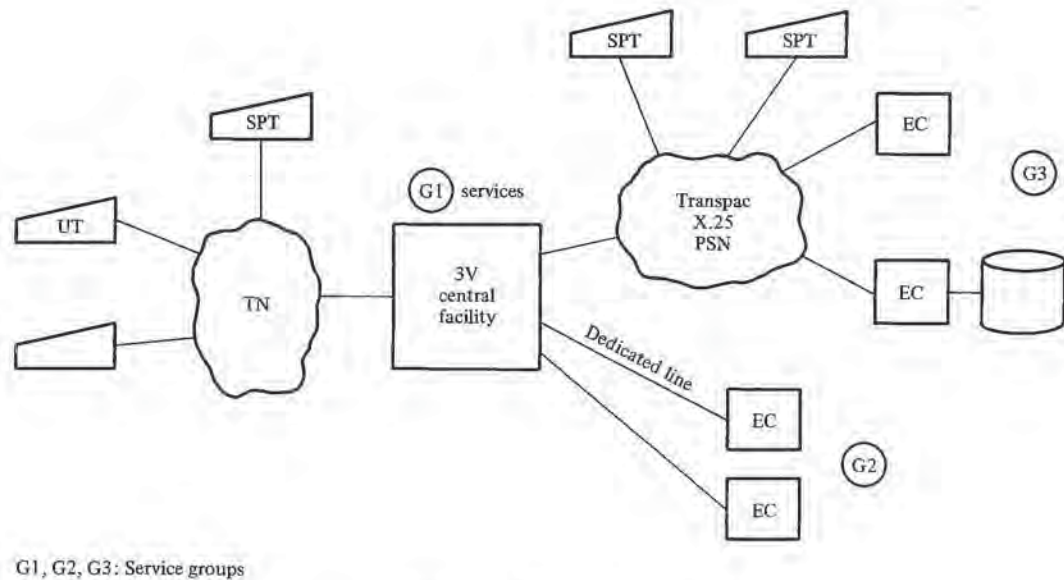
Figure 6.11 Télétel 3V network.
