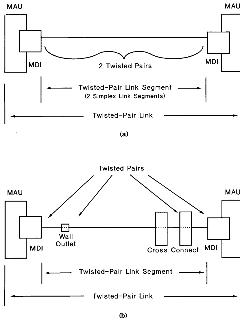
Figure 14-2—Twisted-pair link
