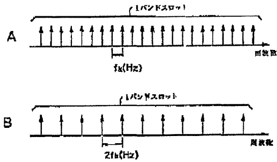
サブキャリアの配列例
