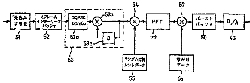
エンコーダの構成
