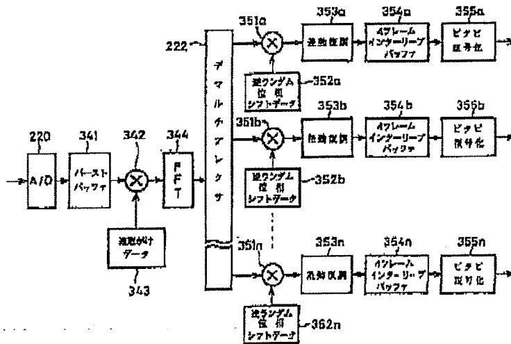
基地局の受信処理
