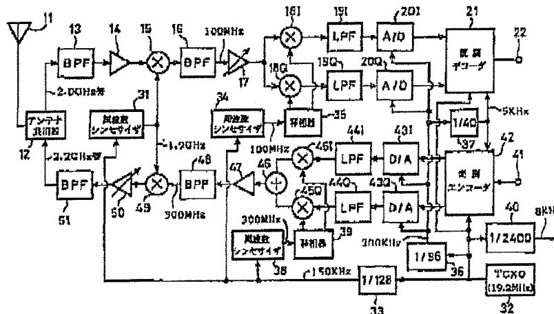
地 本 受 信 の 構 成
