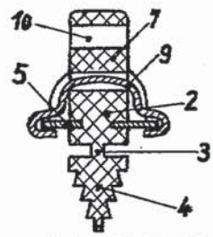
Schnitt B-B
