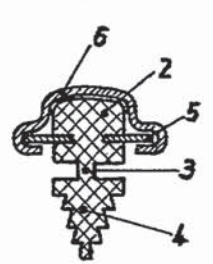
Schnitt C-C
