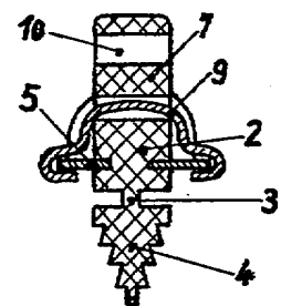
Schnitt B-B
