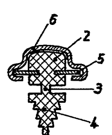
Schnitt C-C
