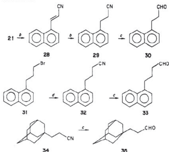
Scheme VI
