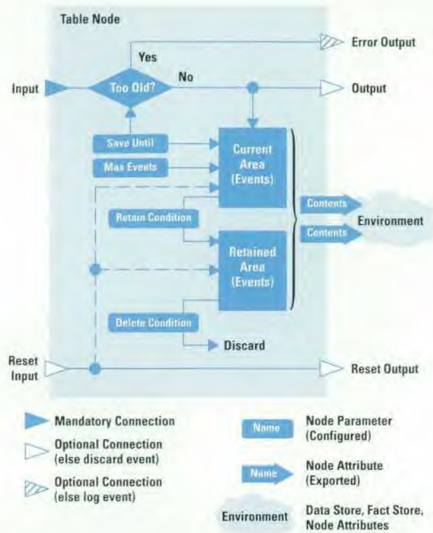
Fig. 1. Table node.
