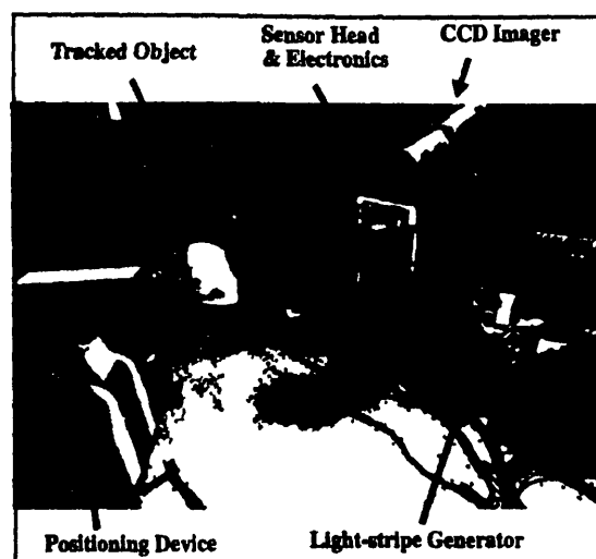
Fig. 4 Pose tracking apparatus
