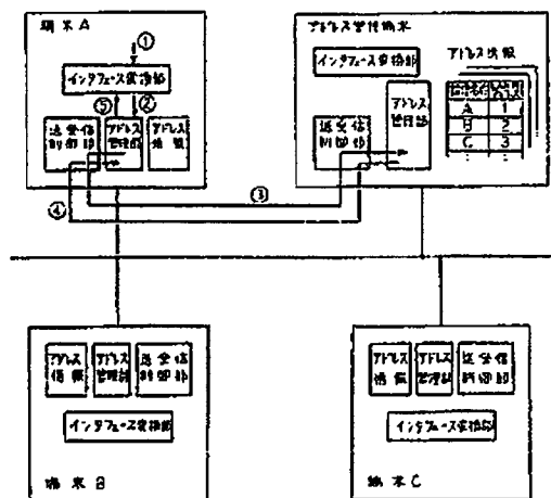
本発明の別実施例の説明図
