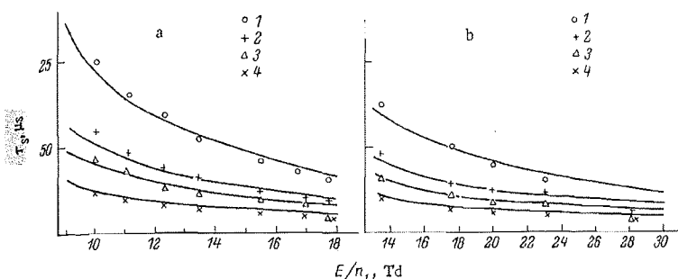
FIG. 4. Curves for \tau_s vs. E/n_1 for a discharge in krypton; p = 10.5 (a) and 6 torr (b). a: 1) n_{e0} = 4 \cdot 10^{10} cm ^{-3} ; 2) 10^{11} ; 3) 1.5 \cdot 10^{11} ; 4) 3.3 \cdot 10^{11} ; b: 1) 3.5 \cdot 10^{10} ; 2) 9.5 \cdot 10^{10} ; 3) 1.6 \cdot 10^{11} ; 4) 3.2 \cdot 10^{11} .
