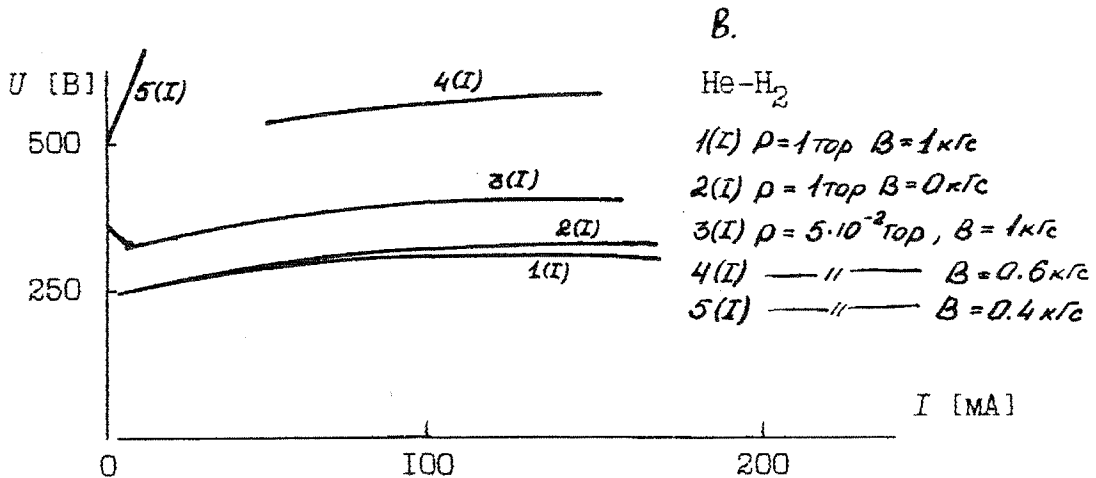
Рис.3.1 Вольт-амперные характеристики стационарного разряда.
