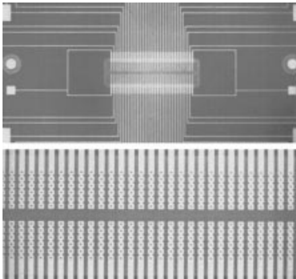
Fig. 3. MARS variable-reflectivity strip mirror.
