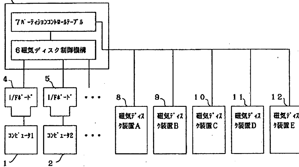
3 磁気ディスク共有装置
