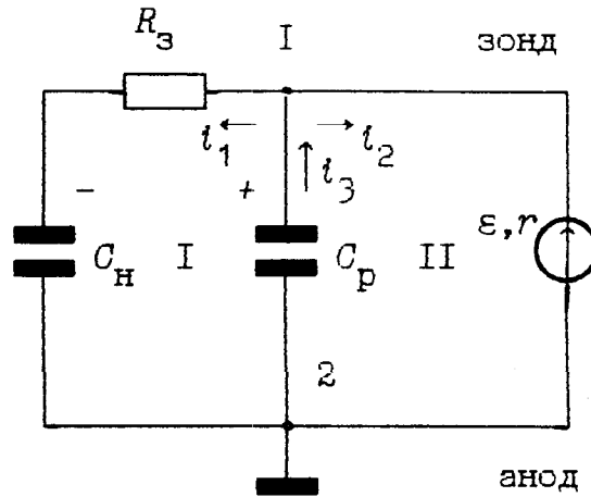
Рис.2.13 Эквивалентная схема генератора развертки при регистрации электронной части зондовой характеристики.
