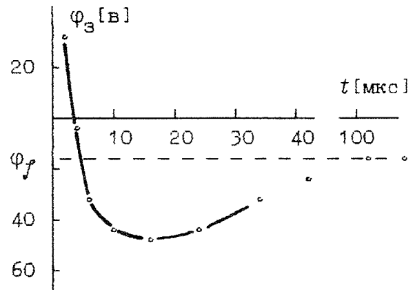
Рис.2.15 Напряжение развертки зонда; • - расчет - - эксперимент
