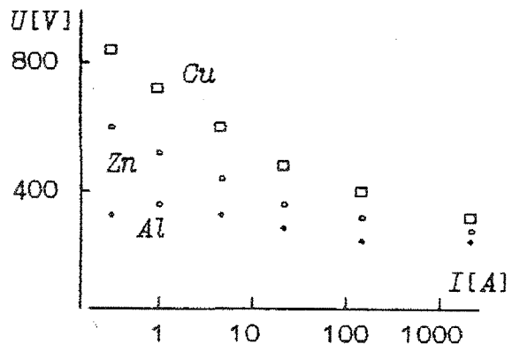
Рис.1.8 Сильноточный режим разряда [63].
