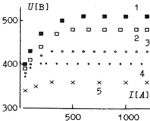
Рис.1.9 Сильноточный (а) и высоковольтный (б) режимы [64-66]. а. I -Ar, p=2 \cdot 10^{-2} тор, 1-B=670 Гц, 2-B=1360 Гц, 3-B=1800 Гц, 4,5- N_2 , H_2 , б. He p=1 \cdot 10^{-3} тор, 1-B=1360 Гц, 2-B=910 Гц, 3-B=670 Гц,
