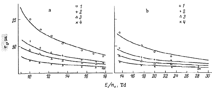
FIG. 4. Curves for \tau_s vs. E/n_1 for a discharge in krypton; p = 10.5 (a) and 8 torr (b). a: 1) n_{e0} = 4 \cdot 10^{10} \text{ cm}^{-3} ; 2) 10^{11} ; 3) 1.5 \cdot 10^{11} ; 4) 3.3 \cdot 10^{11} ; b: 1) 3.5 \cdot 10^{10} ; 2) 9.5 \cdot 10^{10} ; 3) 1.6 \cdot 10^{11} ; 4) 3.2 \cdot 10^{11} .
