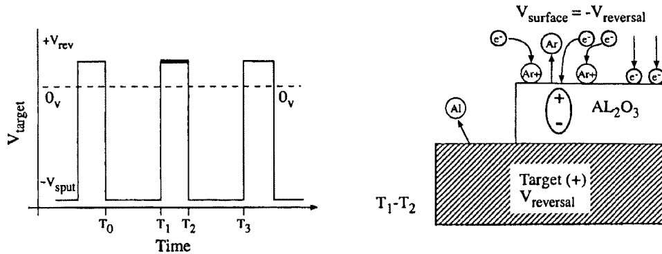
Fig. 3. Reversal mode.
